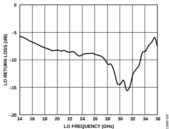
Figure 28. LO Return Loss vs. LO Frequency LO = 13 dBm
