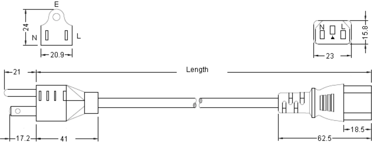
Dimensions : Millimetres
