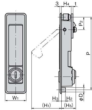
A-1230-A-1-1
