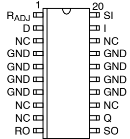
SO-20L
