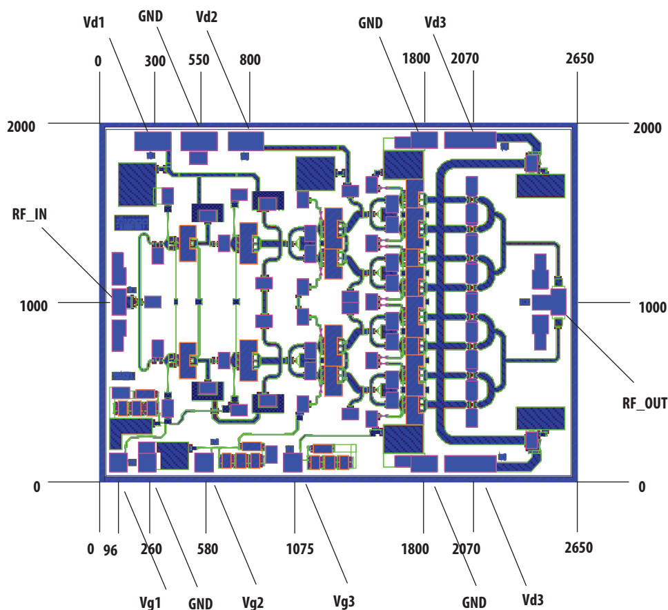
Figure 15. Die dimensions
