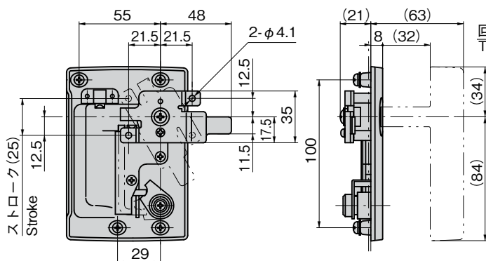
ハンドル開閉角度90° Handle opening/closing angle
