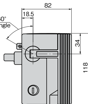
止め金固定ギア Stopper plate fixed gear
