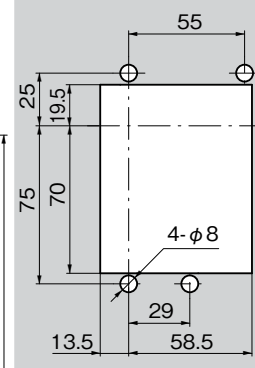
パネル穴明け寸法 Panel drilling dimensions
