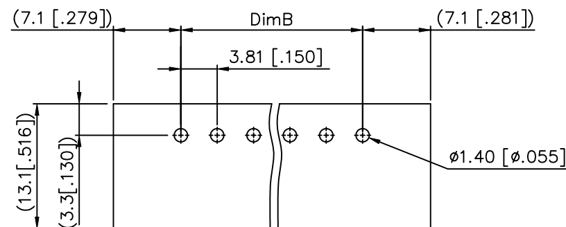
P.C.B LAYOUT
