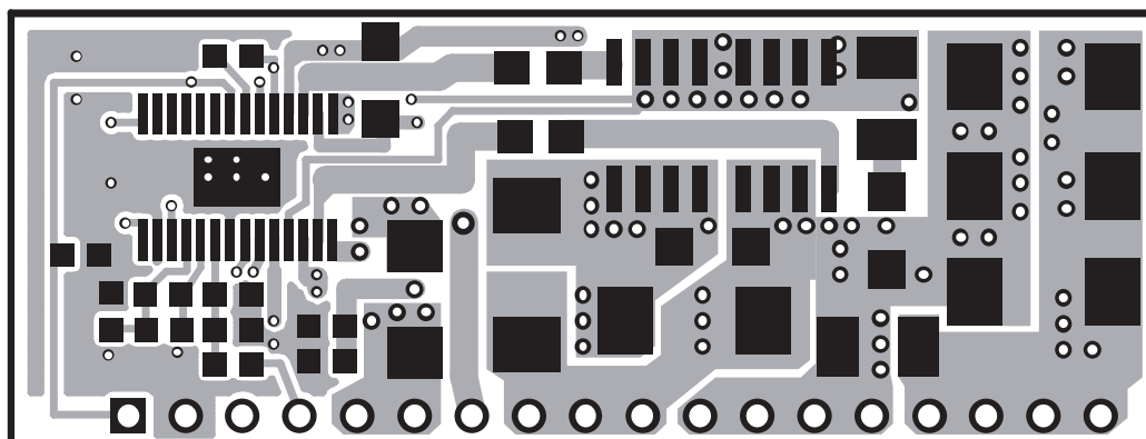
Top Layer
