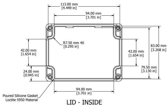
LID - INSIDE
