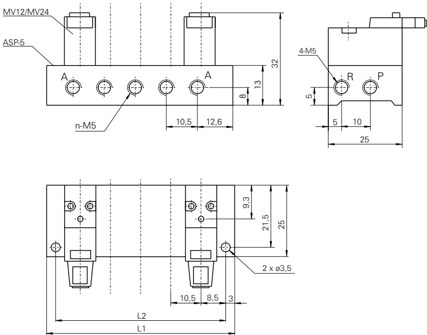
Mehrfachanschlussplatte (ASP-2...-10)
