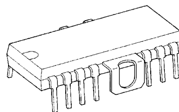
HDIP14-P-500-2.54A
