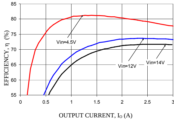
V_o = 0.6V
