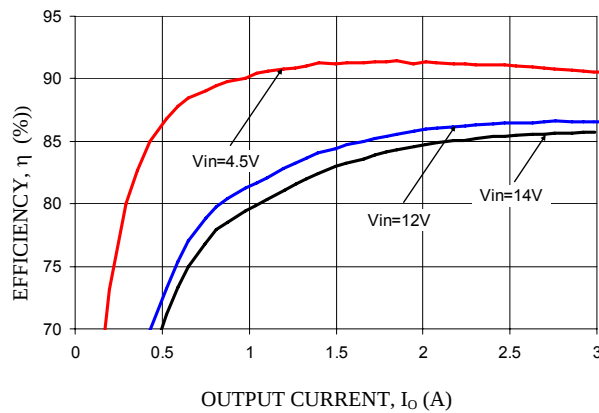
V_o = 1.8V
