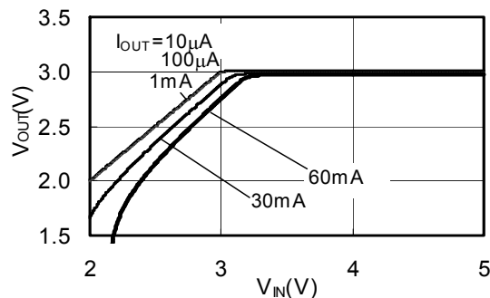
S-818A30A ( T_a=25^\circ\text{C} )
