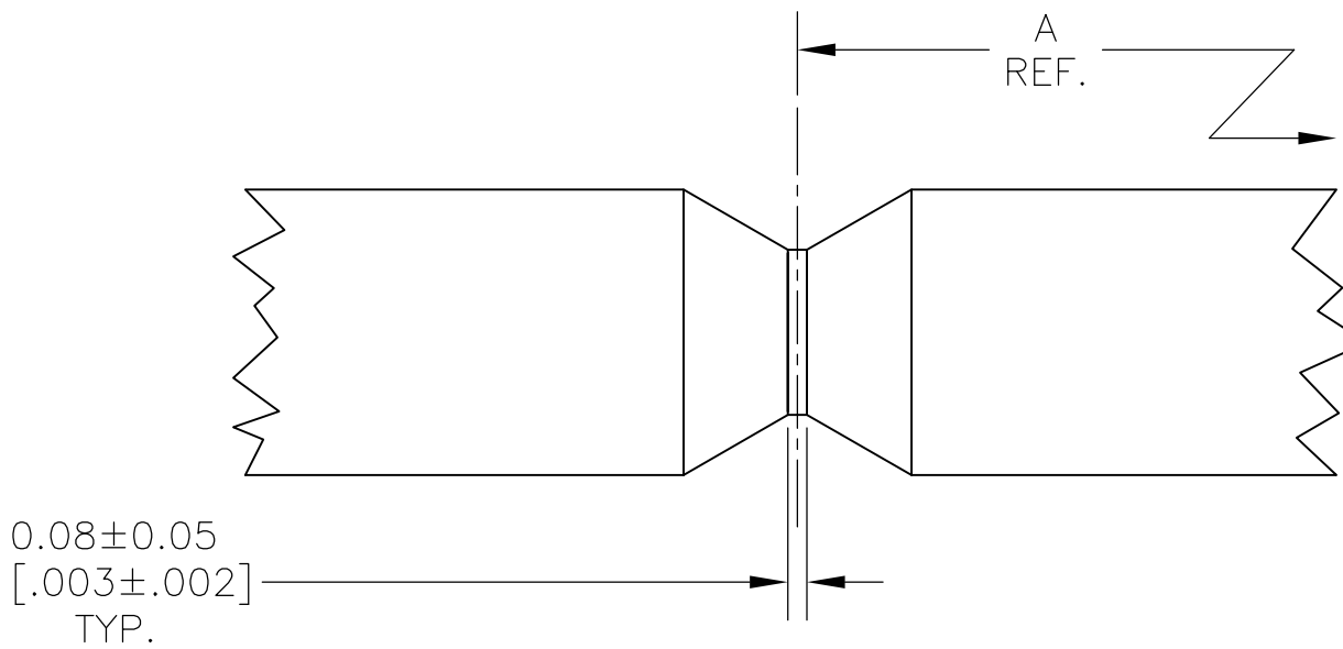
DETAIL W 30:1
