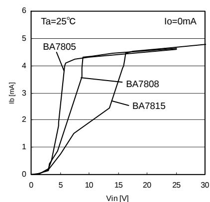
Fig.16 V_{in} - I_b
