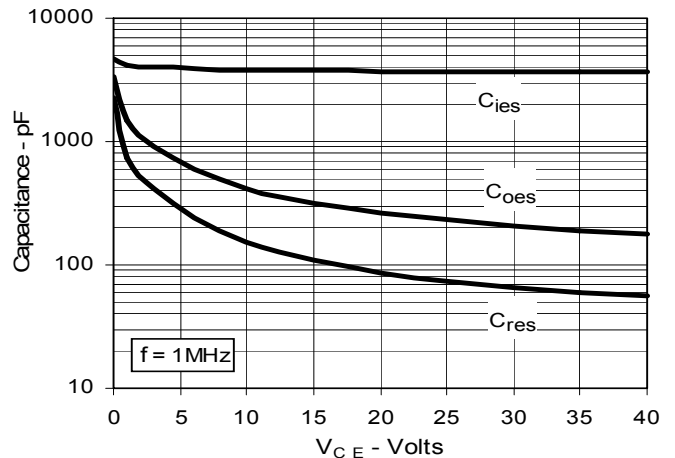
Fig. 12. Capacitance
