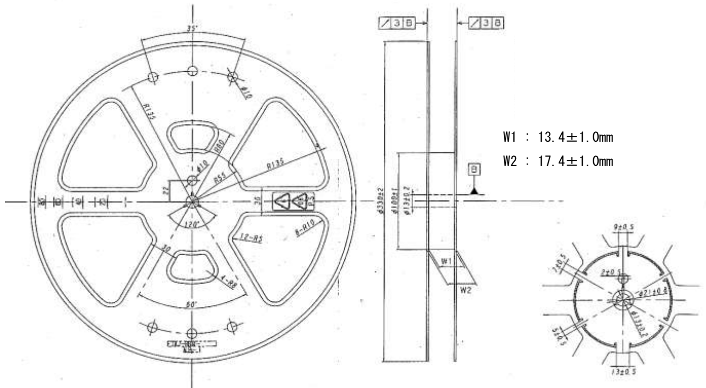
図9 リール寸法
