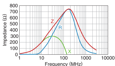
MPZ1608S601A
