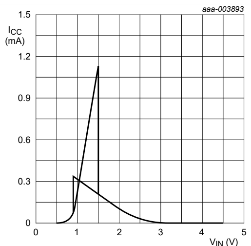
a. V_{CC} = 4.5\text{ V}
