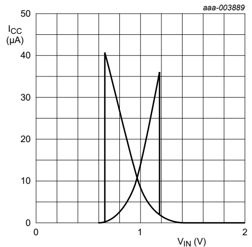
a. V_{CC} = 2.0\text{ V}
