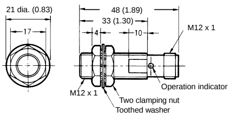
Fig. 16: E2E-X5E□-M1/F□-M1-N
