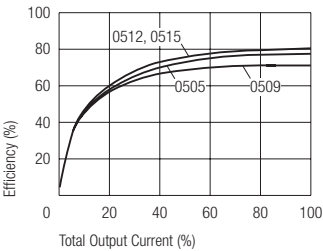
R05A/Bxx
