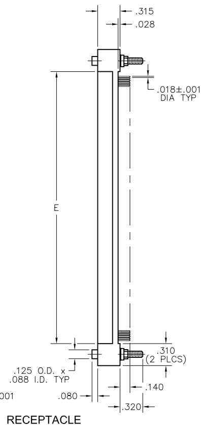
RECEPTACLE
