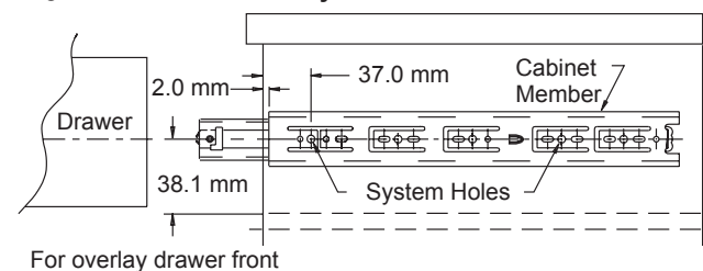
Figure 2 32 mm System—Cabinet
