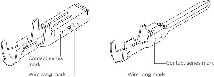
Receptacle Contact
