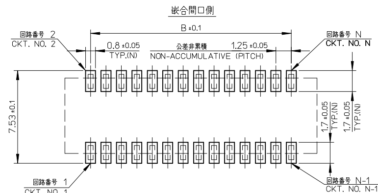
推奨基板レイアウト
