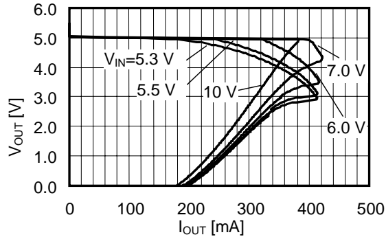
S-L2980A50 (Ta=25°C)
