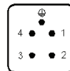
Receptacle
