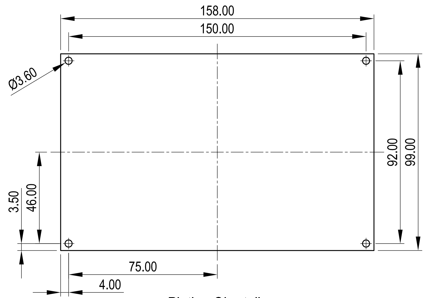
Platine Oberteil PCB top part
