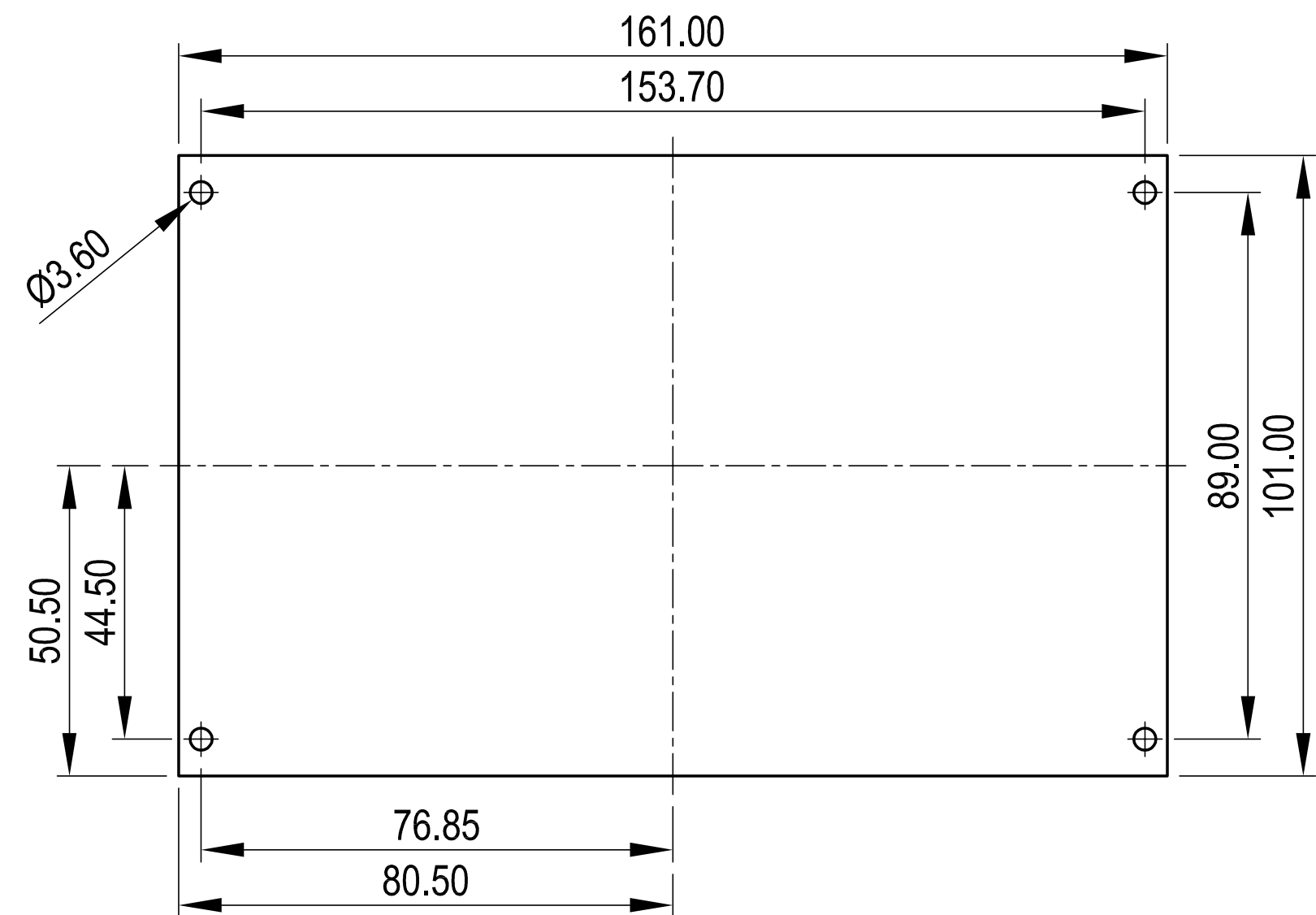
Platine Unterteil PCB base part
