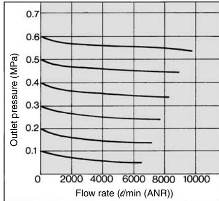
AR825 R_c 1 \frac{1}{2}
