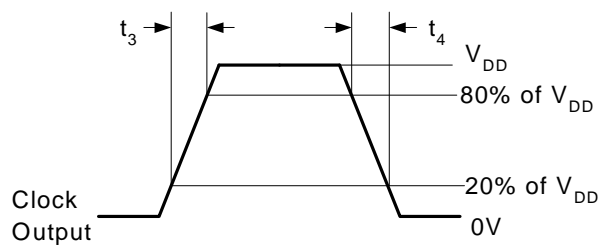
Figure 11. ER = (0.6 \times V_{DD})/t_3 , EF = (0.6 \times V_{DD})/t_4
