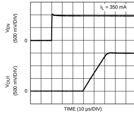
1.5-V Option
