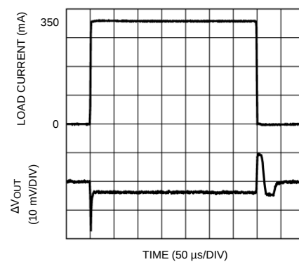
1.5-V Option
