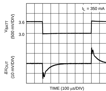
1.5-V Option
