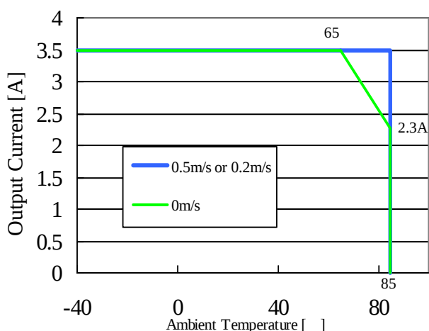
MPD6D103S ( V_o=1.5\text{V} )
