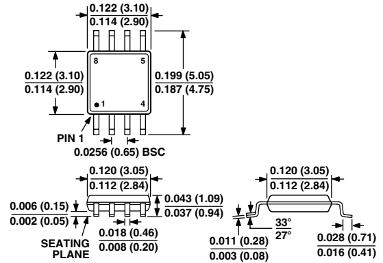
8-Lead MINI SOIC (RM-8)
