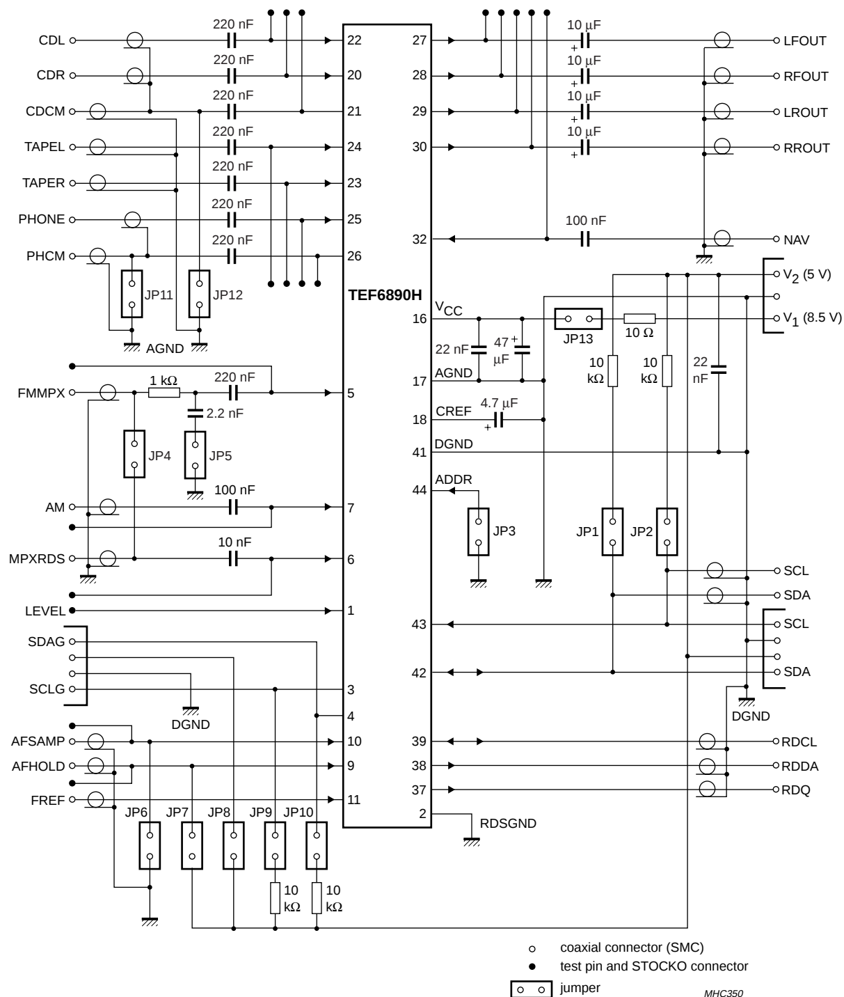
Fig.23 Test circuit.
