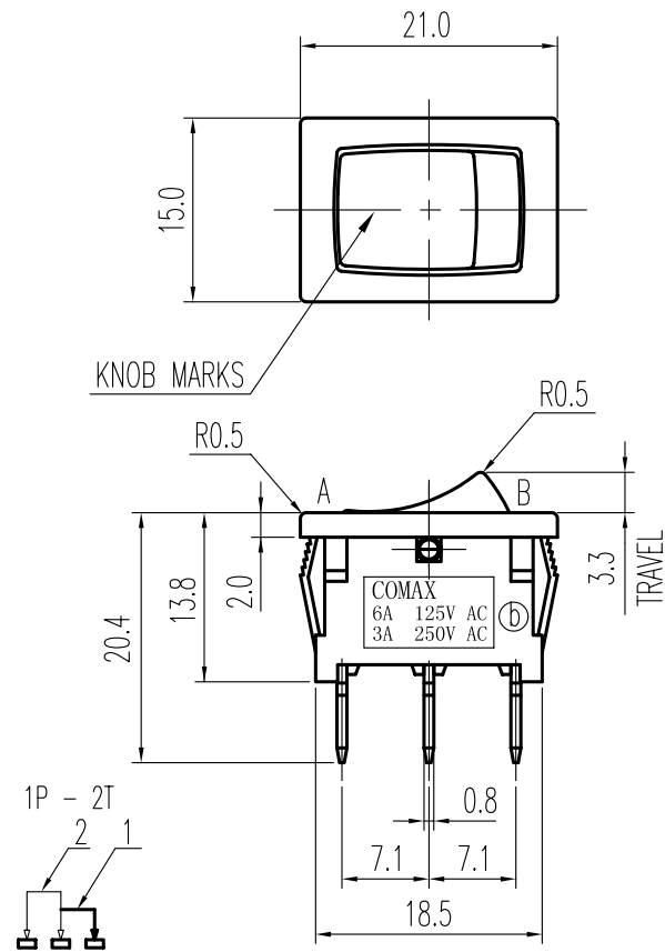
示意图 SCHEMATIC
