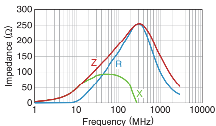
MMZ2012S102A
