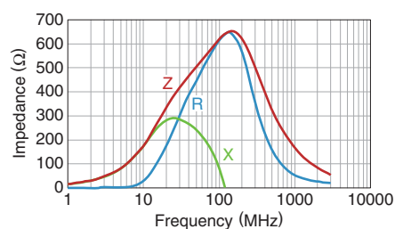
MMZ2012S601A
