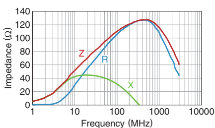
MMZ2012R102A
