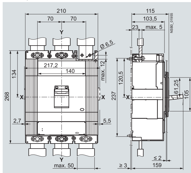
3RV10 83, 3RV13 83
