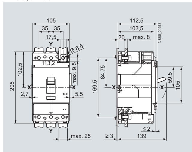
3RV10 83, 3RV13 83
