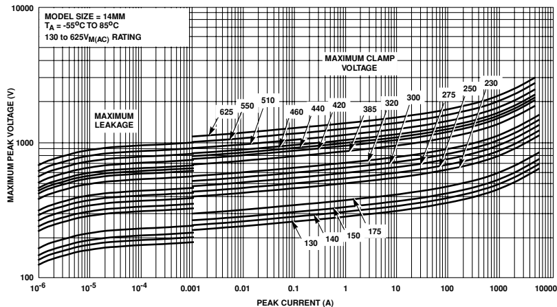
V14E130(P) - V14E625(P)
