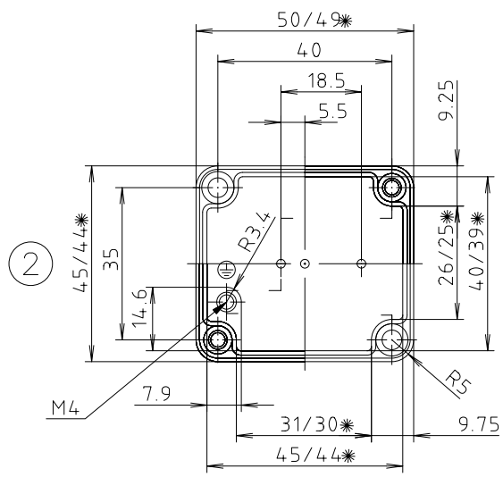
Unterteil
