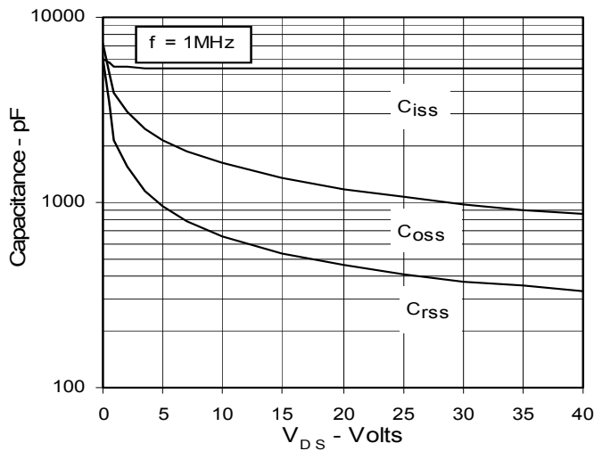
Fig. 11. Capacitance
