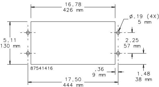
CUTOUT DIMENSIONS
