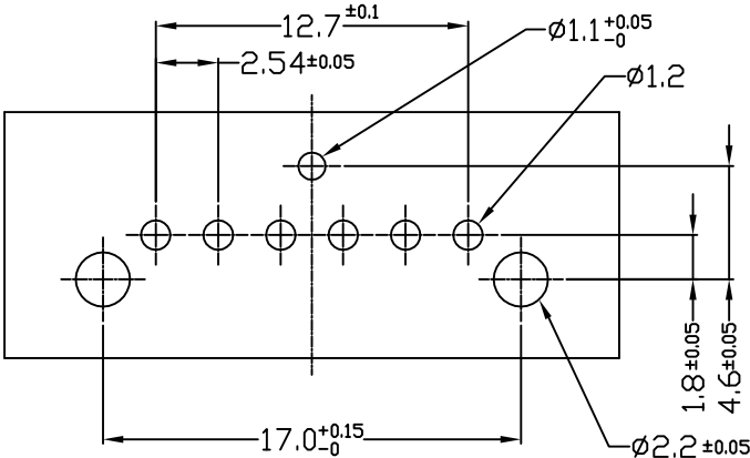
P.C.B LAYOUT-REF
