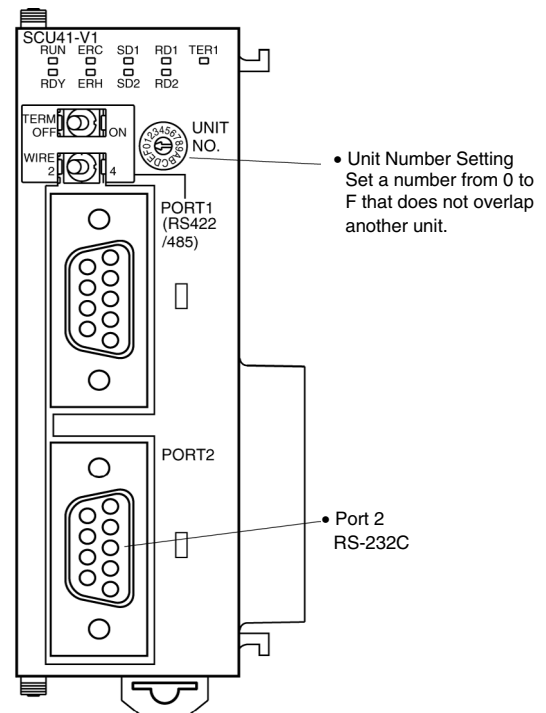
CJ1W-SCU41-V1
