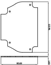
BOTTOM-PCB
