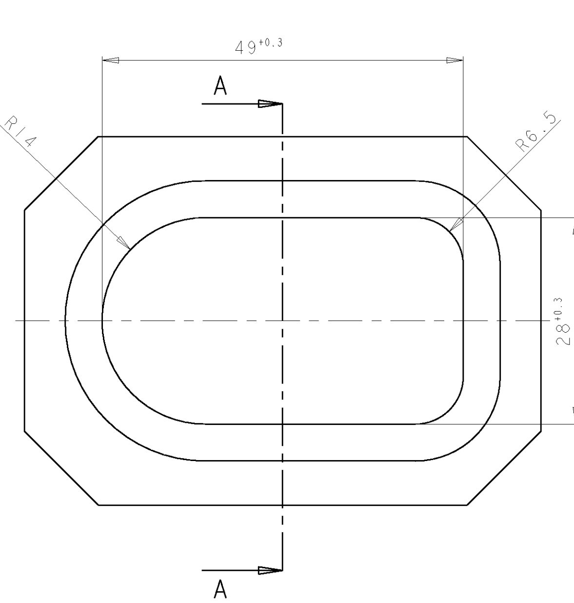
CUT OFF Befestigungsausschnitt
