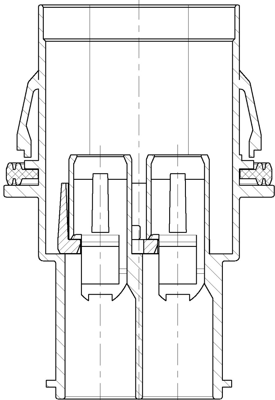
SECONDARY LOCKING IN LOCKED POSITION (SLIDING DISTANCE: 2.5MM) Zweite Kontaktsicherung in Endraststellung (Verschiebeweg: 2.5mm)
