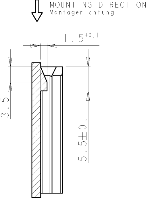
SECTION A-A Schnitt
