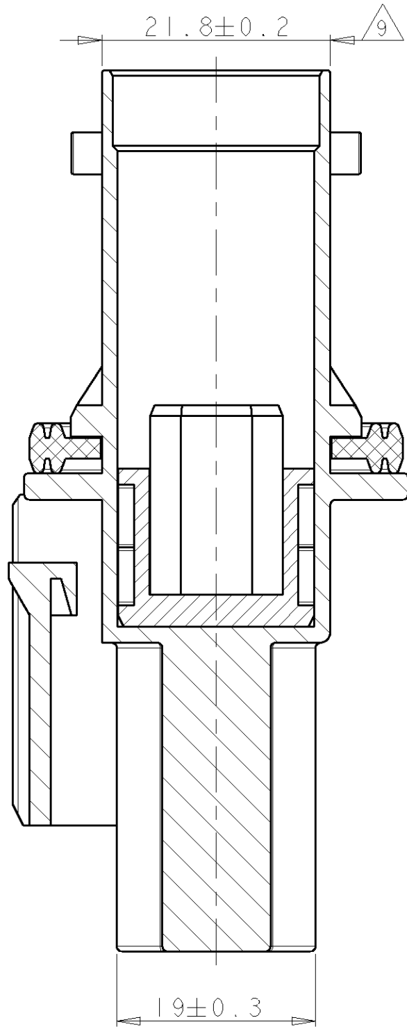
SECONDARY LOCKING IN PRE-LOCKED POSITION Zweite Kontaktsicherung in Vorraststellung
