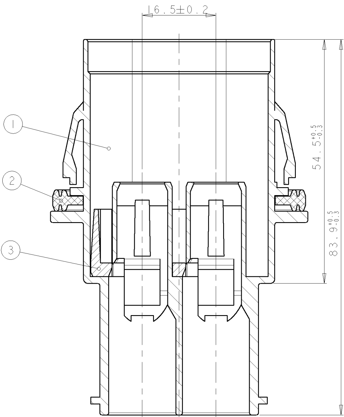
SECONDARY LOCKING IN PRE-LOCKED POSITION Zweite Kontaktsicherung in Vorraststellung
