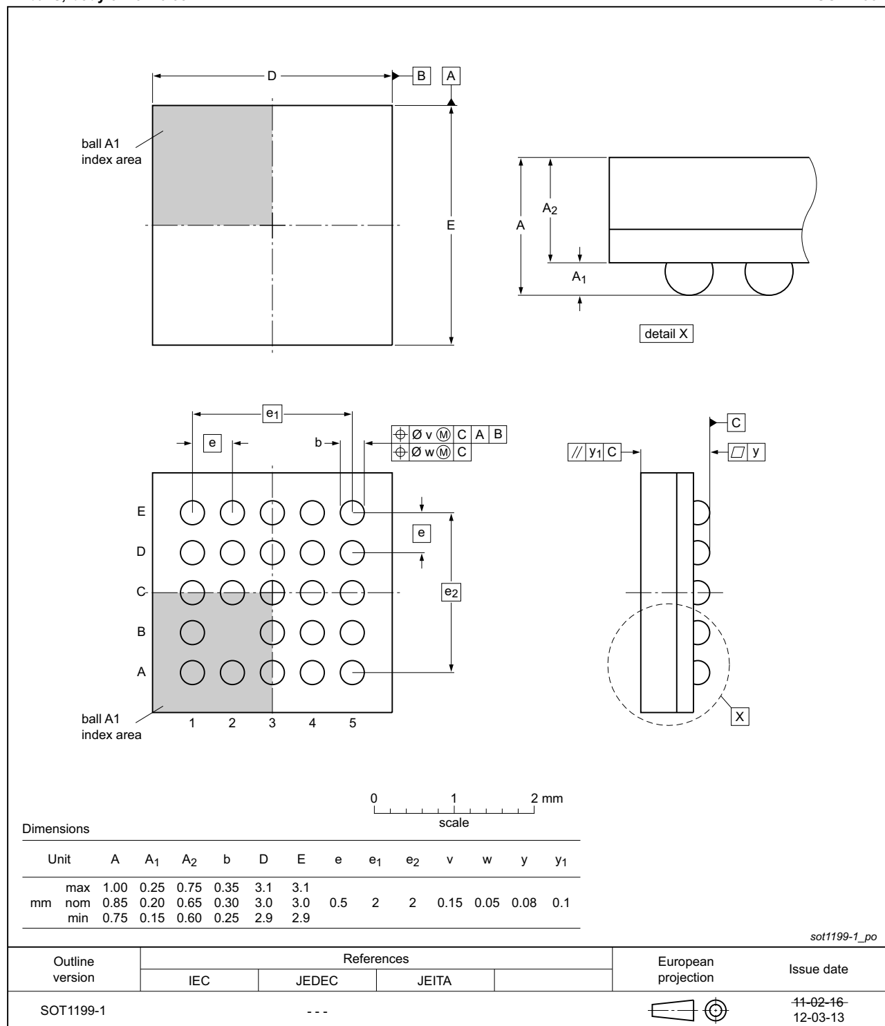
Fig 41. Package outline SOT1199-1 (VFPGA24)
