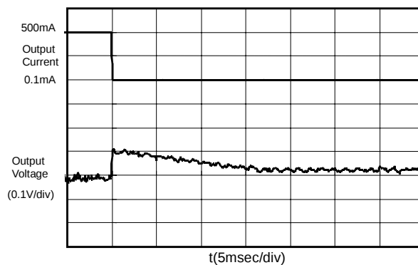
S-8521C30MC (Vin:3.6V)
