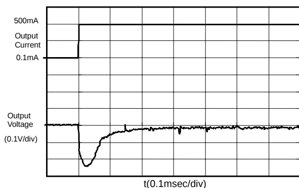
S-8520C30MC (Vin:3.6V)
