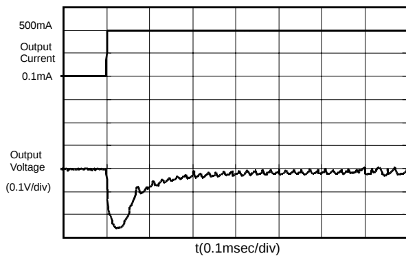
S-8521C30MC (Vin:3.6V)
