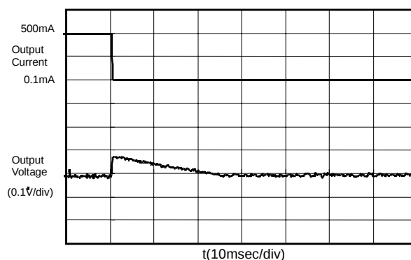
S-8520C30MC (Vin:3.6V)
