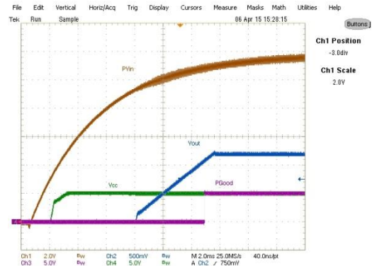
Fig. 3: P_{Vin} Start up at 25A Load Ch 1 : P_{Vin} , Ch 2 : V_{out} , Ch 3 : P_{Good} , Ch 4 : V_{cc}
