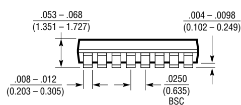
GN16 (SSOP) 0502
