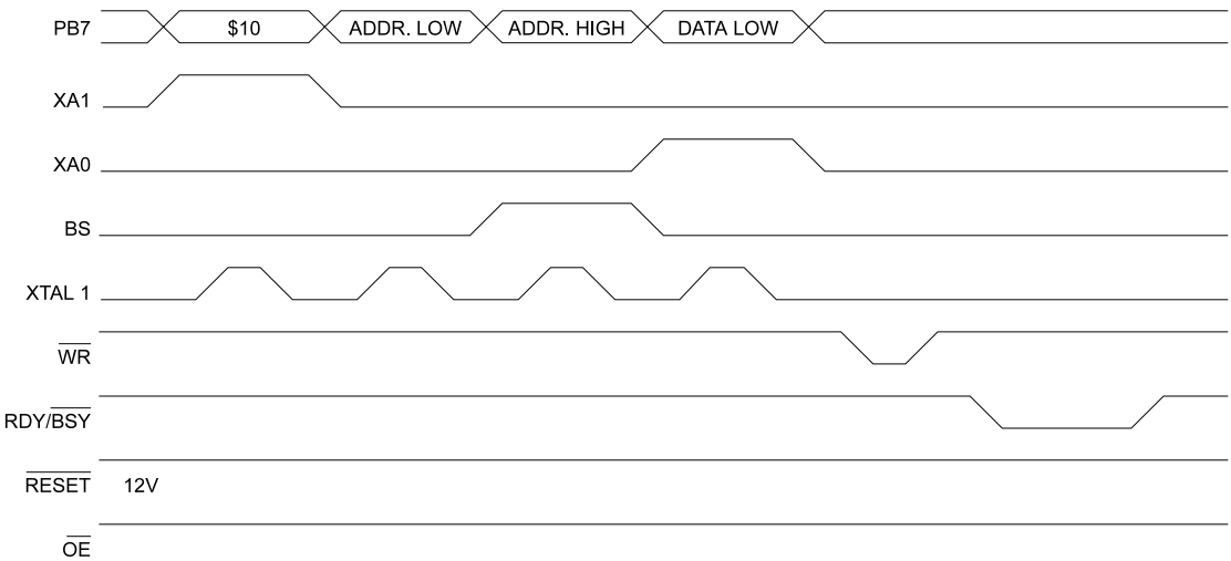
图 32 编程波形二
