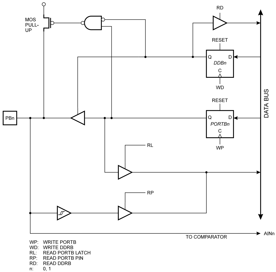
图 23 B 口示意图 (PB2、PB3 和 PB4)
