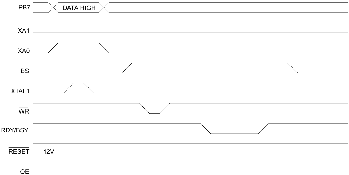
图 32 编程波形二
