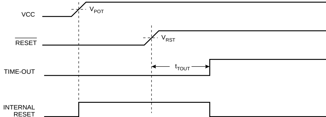
图 15 MCU 启动， \overline{\text{RESET}} 由外电路控制
